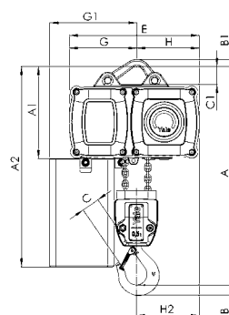
CPV/CPVF mit Tragbügel, 500 - 5.000 kg, zweisträngig
