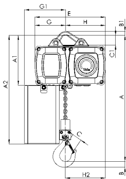
CPV/CPVF mit Tragbügel, 125 - 2.500 kg, einsträngig
