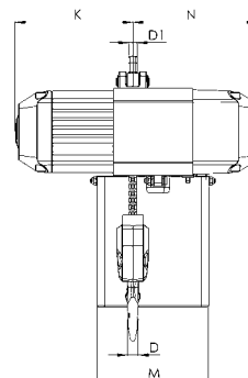
CPV/CPVF mit Tragbügel, 500 - 5.000 kg, zweisträngig
