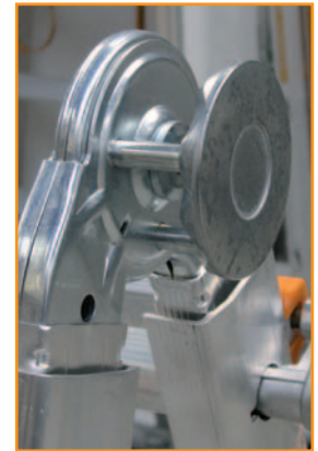
Entsperrtes Gelenk
