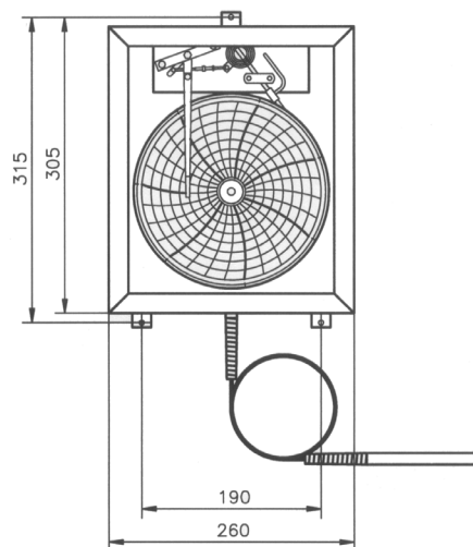
Bild 7 Kreisblattschreiber Typ 355
