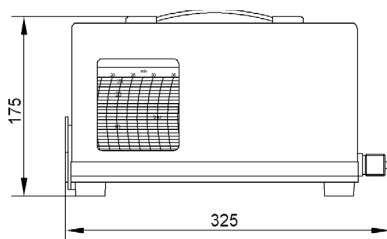
Bild 6 Trommelschreiber Typ 354
