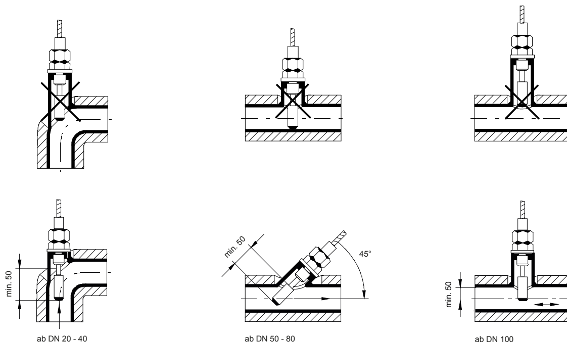
Bild 9 Fühlereinbau
