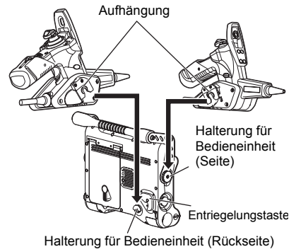
Anbringung hinten: Zum Transport
