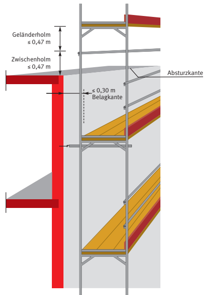
Bild 23: Gerüst mit innen liegender Absturzsicherung
