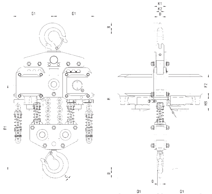
Modell CPA ATEX mit Traghaken, viersträngig 10.000 kg
