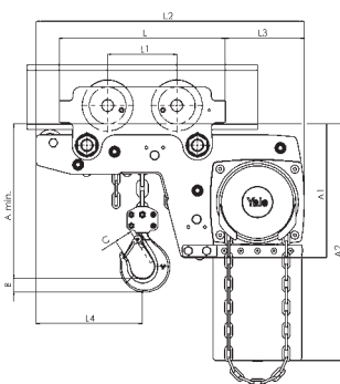
Modell Yalelift LHG ATEX, einsträngig 500 - 3.000 kg
