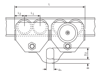
Modell HTG ATEX 20.000 kg
