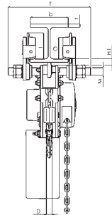
Modell Yalelift LHP ATEX, einsträngig 500 - 3.000 kg
