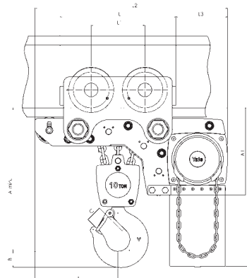
Modell Yalelift LHG ATEX, dreisträngig 10.000 kg
