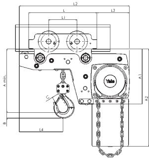
Modell Yalelift LHP ATEX, einsträngig 500 - 3.000 kg
