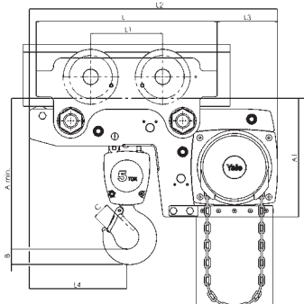
Modell Yalelift LHP/LHG ATEX, zweisträngig 5.000 kg
