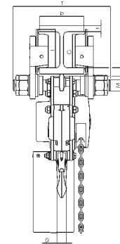
Modell Yalelift LHP/LHG ATEX, zweisträngig 5.000 kg
