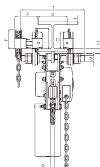
Modell Yalelift LHG ATEX, einsträngig 500 - 3.000 kg
