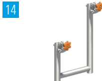
1323.180 Fahrbalken mit Bügel Stahl-Rechteckrohr, feuerverzinkt, zur Basisverbreiterung für Gerüste
