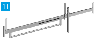
1338.320 Fahrbalken mit 2 Rohrverbindern, verstellbar Stahl-Rechteckrohr, feuerverzinkt. Zur Basisverbreiterung für fahrbare Sonderaufbauten. Systemauf- bauten nur in Verbindung mit Art.-Nr. 1337.000 möglich
