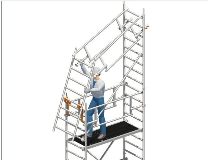
1. Aufstecken der ersten Standleiter. Anbringen der Uni Montagehaken und Positionierung der zweiten Standleiter zur Montage des Doppelgeländers auf beiden Seiten.
