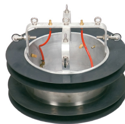
FORMIER-VORRICHTUNGEN
