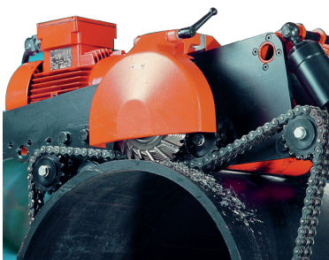
ROHR-UMLAUFSAGEN
