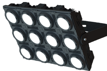
BAUSTELLENBELEUCHTUNGEN
