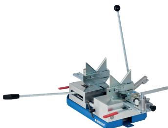
STUMPSCHWEISSGERÄT
